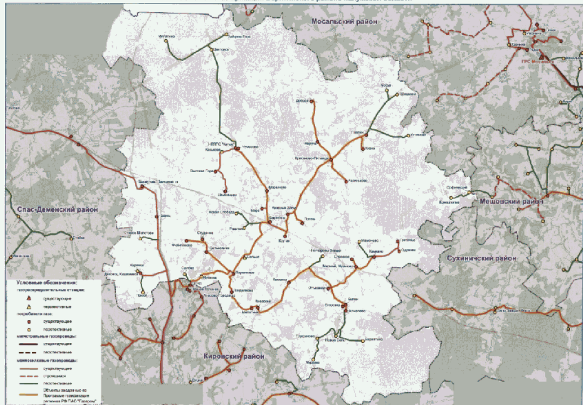
Схема газоснабжения и газификации Бярытинского района Калужской области
