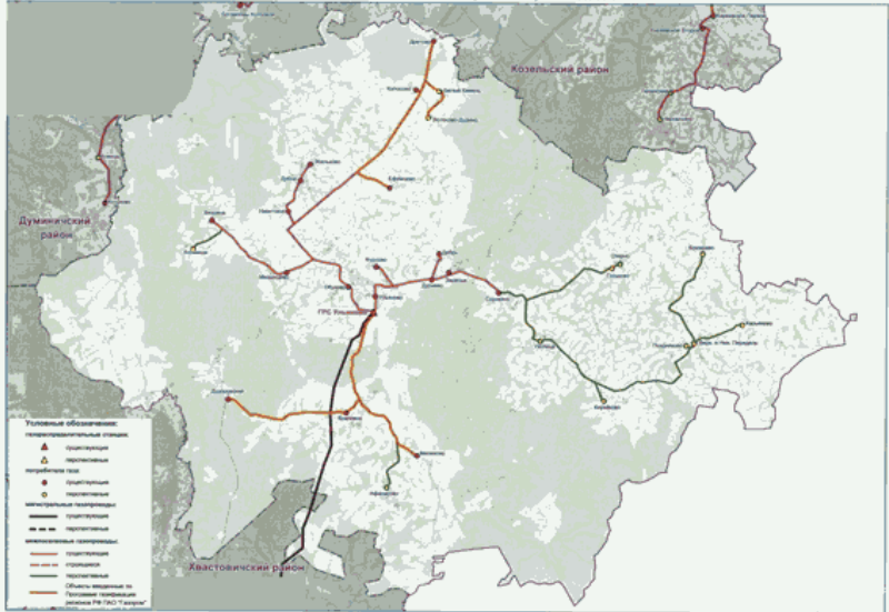
Схема газоснабжения и газификации Ульяновского района Калужской области
