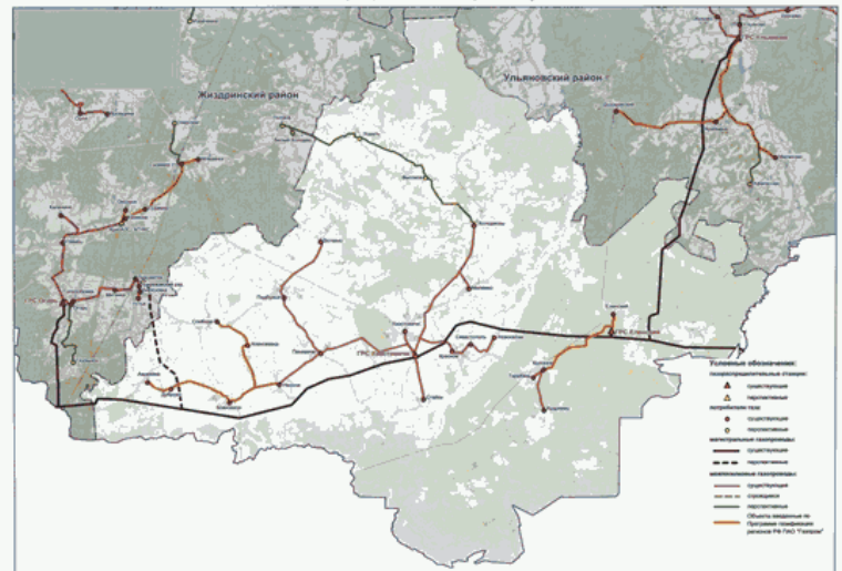
Схема газоснабжения и газификации Хвостовского района Калужской области
