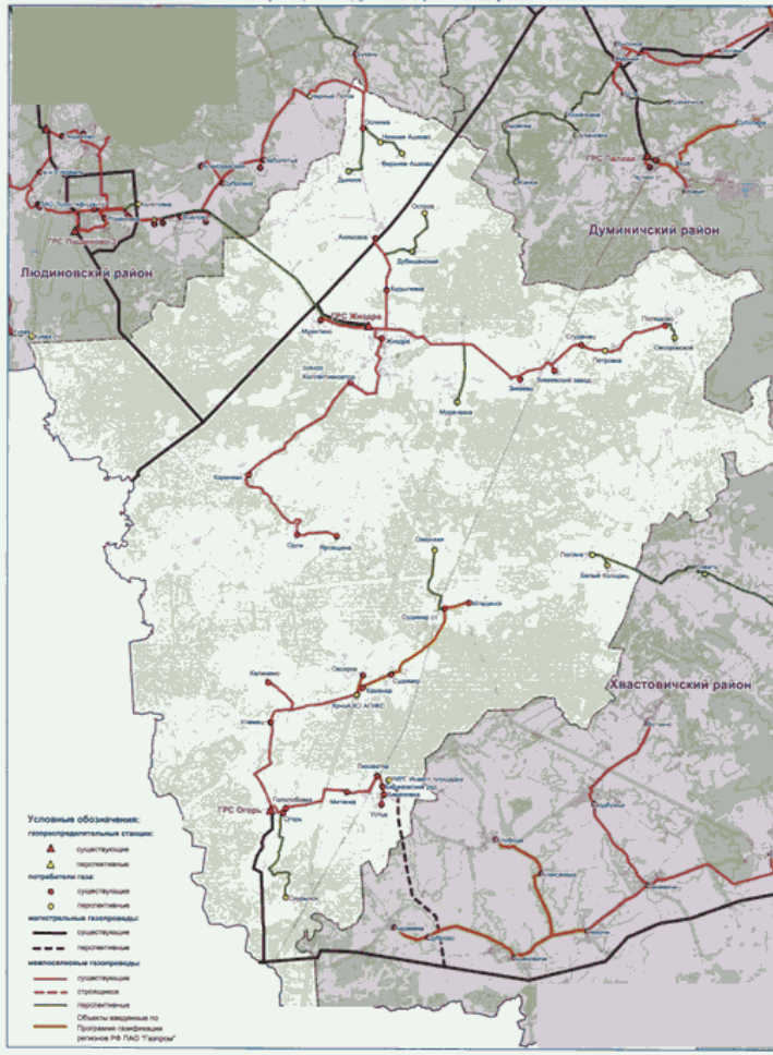
Схема газоснабжения и газификации Жиздрина Калужской области
