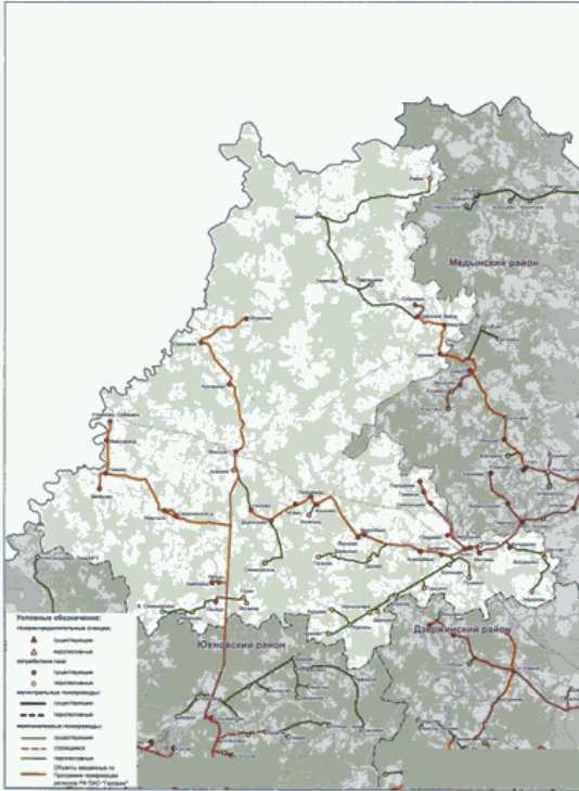
Схема газоснабжения и газификации Износковского района Калужской области
